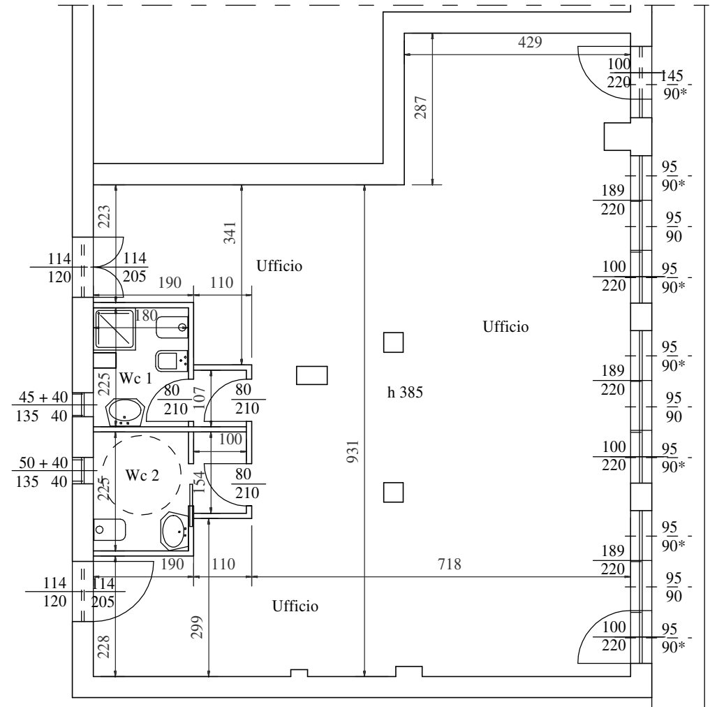
Pianta Piano Terra Stato di Progetto
